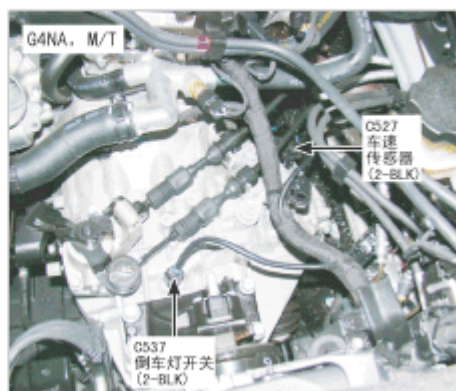
156. 变速器顶部
