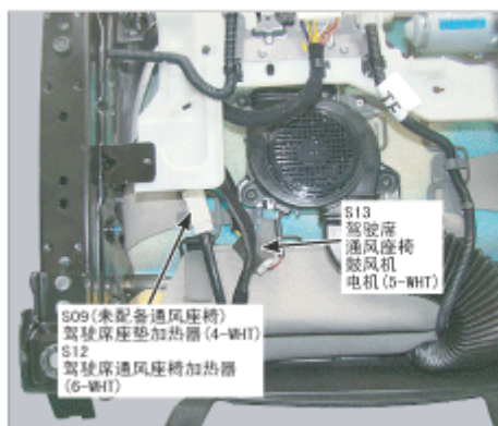
154. 驾驶员座椅
